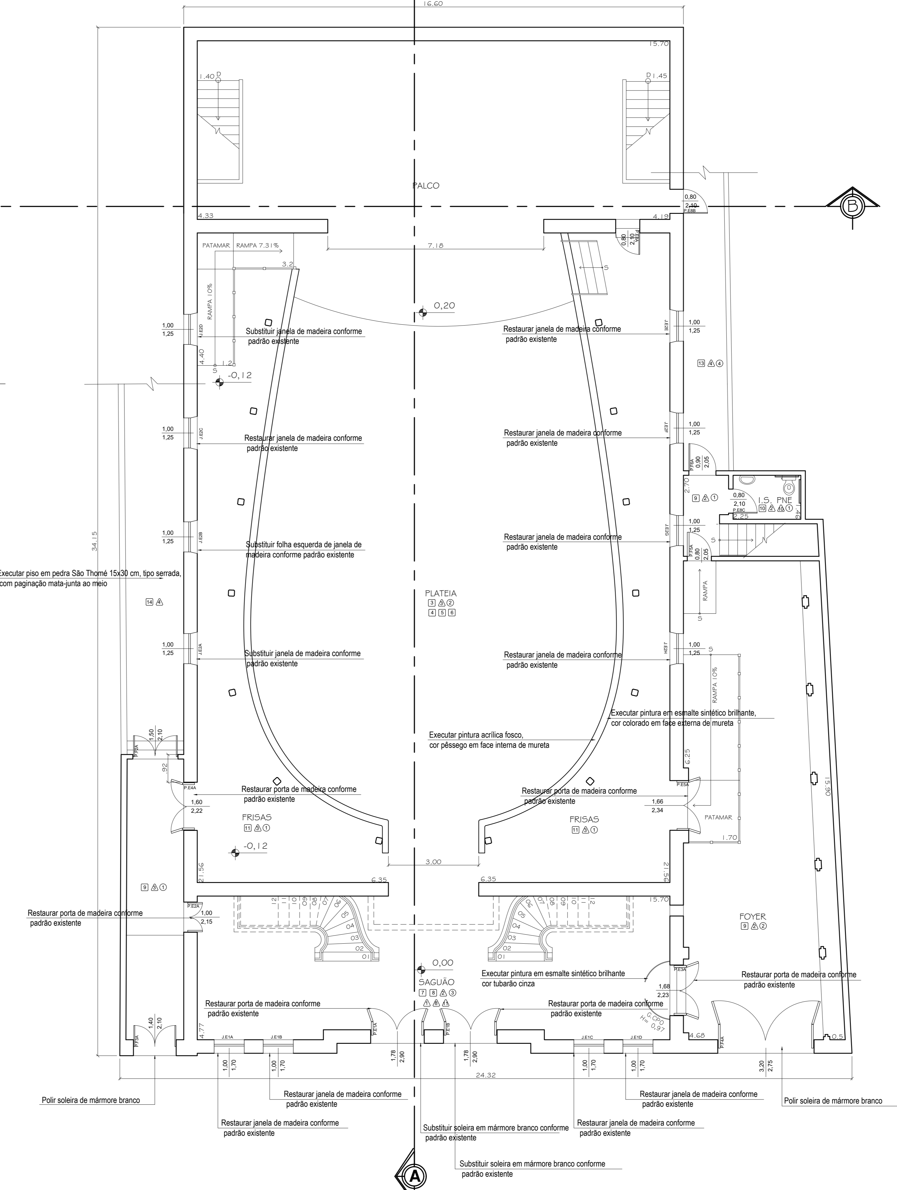
P.B PVTO TERREO AREA ..... 603,62m 2
